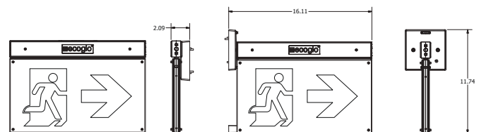
Installation sur le mur
