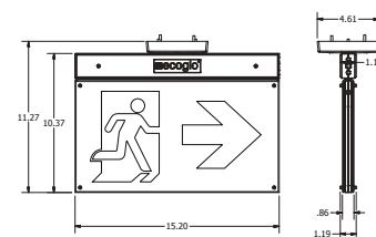
Installation au plafond
