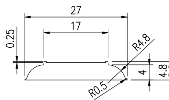
BAR DETAIL SCALE: 1:1
