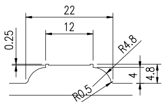
DOME DETAIL SCALE: 1:1
