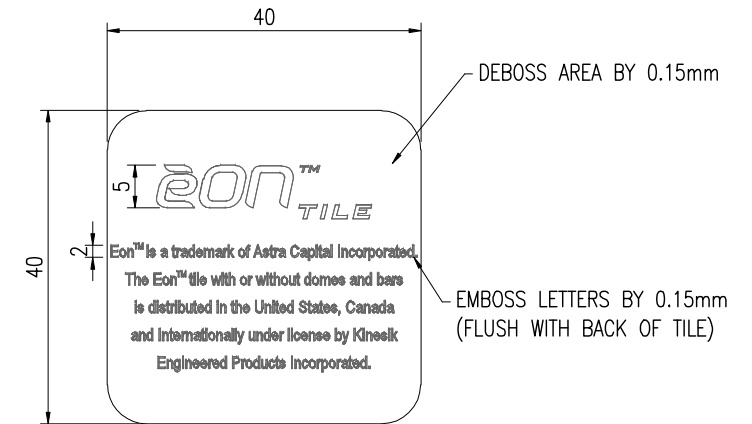
IP INFORMATION SCALE: 1:1
